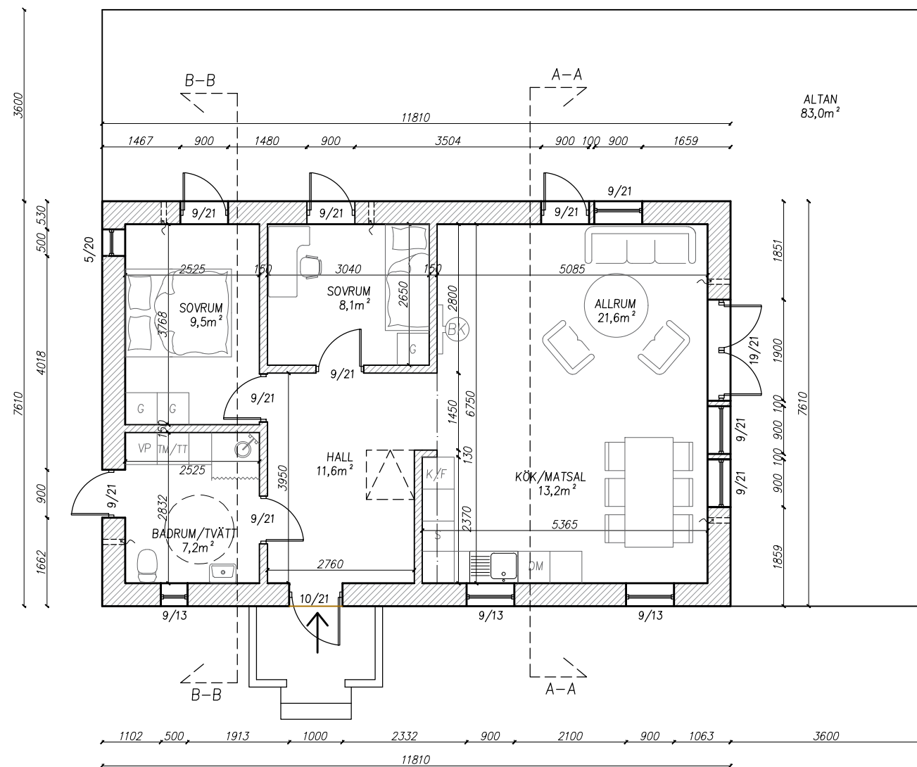
ENTRÉPLAN SKALA 1:100 (A3)
